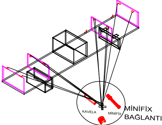
SOL YAN - SOL DİKORTA KERTİKLİ-SAĞ DİKORTA-SAĞ YAN MONTAJ
