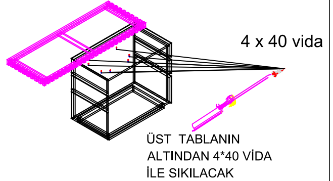
ÜST MERMER TABLA MONTAJ
