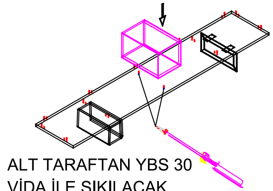
ORTA KUTU MONTAJ
