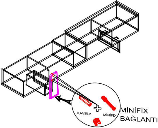
DÖKÜM ÖN KLAPA MONTAJ
