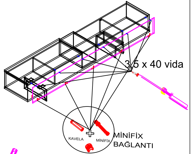
ARKA PARÇA MONTAJ
