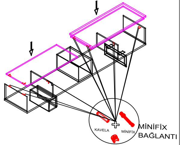
SOL ÜST TABLA-SAĞ DÖKÜM ÜST TABLA MONTAJ
