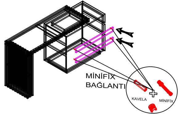
ÇEKMECE ARA KLAPALAR MONTAJ
