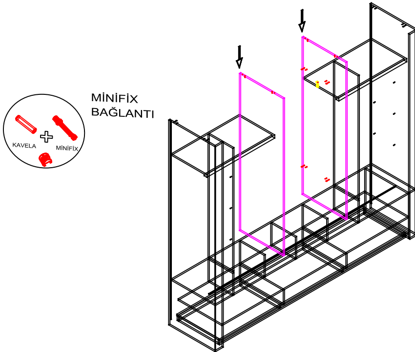
ORTA SAĞ-SOL BÜYÜK DİKORTA MONTAJ
