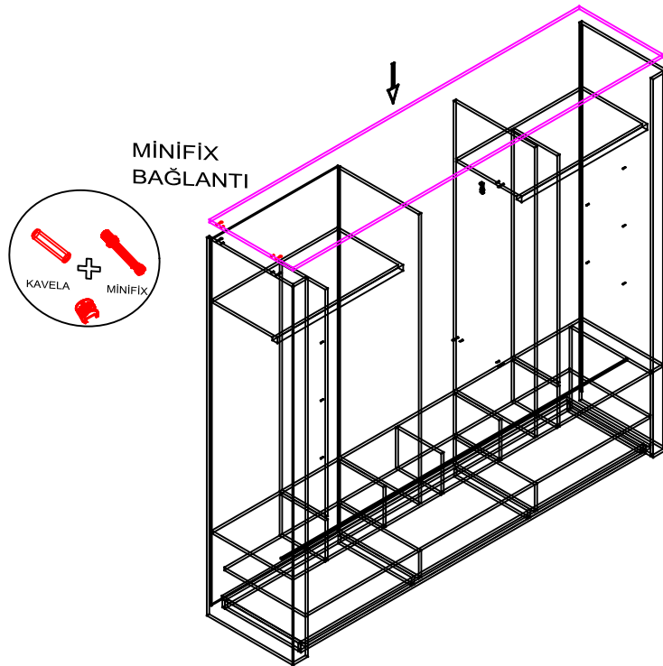
ÜST TABLA MONTAJ
