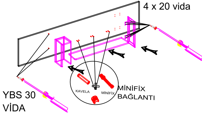
ALT TABLA AYAK-ALT TABLA DESTEK PARÇA MONTAJ
